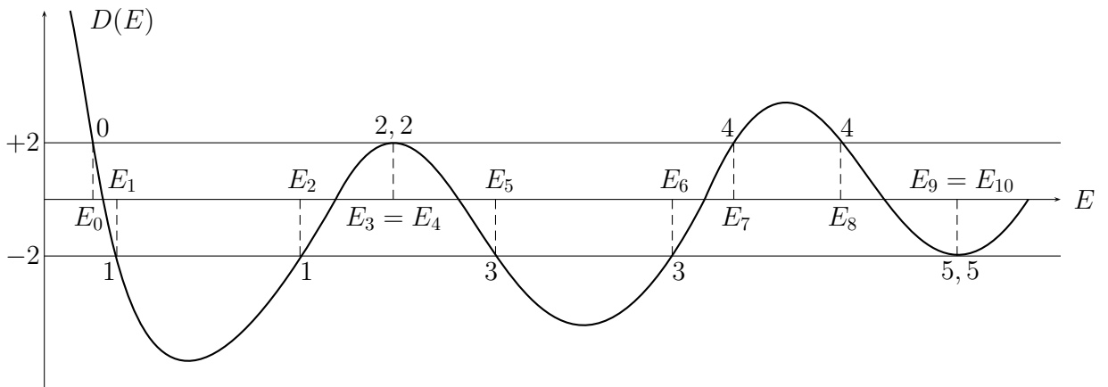
Figura 3.4: Discriminante \mathcal{D}(E) en un caso genérico de un potencial periódico
