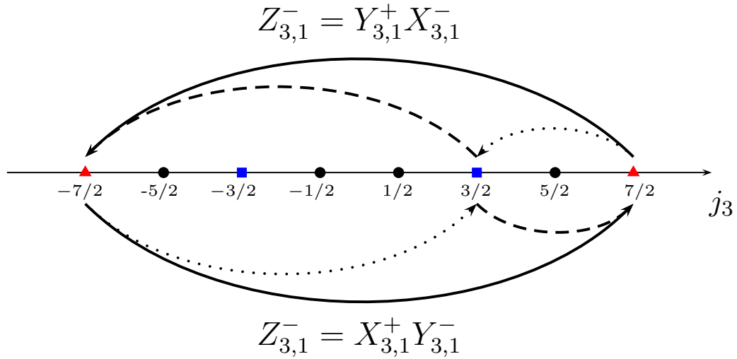
Figura 6.5: Acción de los operadores Z_{3,1}^- en correspondencia con (6.44).
