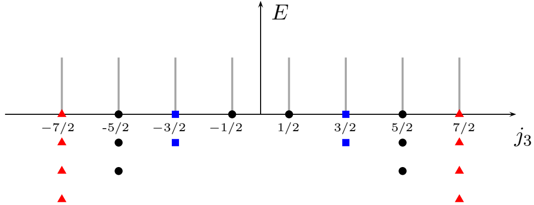
Figura 6.2: Espectro del sistema \text{AdS}_2 con flujo de AB semientero ( \alpha = 1/2 ).
