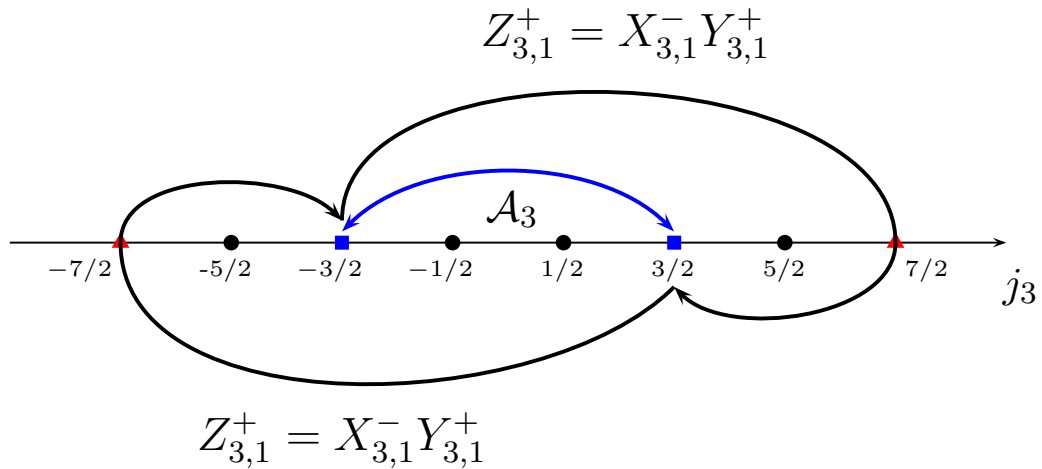
Figura 6.6: Acción de los operadores Z_{3,1}^+ en correspondencia con (6.45).
