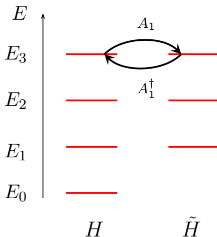
Figura 2.1: Transformación de Darboux generada por un estado base sin nodos de naturaleza no periódica. La energía E_0 esta ausente del espectro de \tilde{H} . Las flechas indican las direcciones en que actúan las transformaciones de Darboux.
