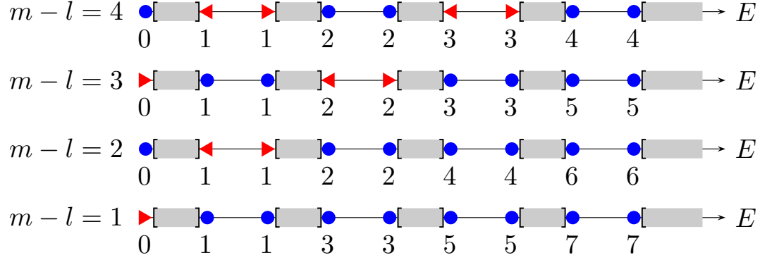
Figura 5.1: Esquema de la estructura de bandas para los sistemas self-isospectrales con m = 4 . Los triángulos (círculos) indican los estados del borde de bandas aniquilados por \mathcal{X}_{m,l}^{\pm} ( \mathcal{Y}_{m,l}^{\pm} ) y los números bajo de ellos indican su número de nodos. Los estados con un número par (impar) de nodos son periódicos (anti-periódicos)
