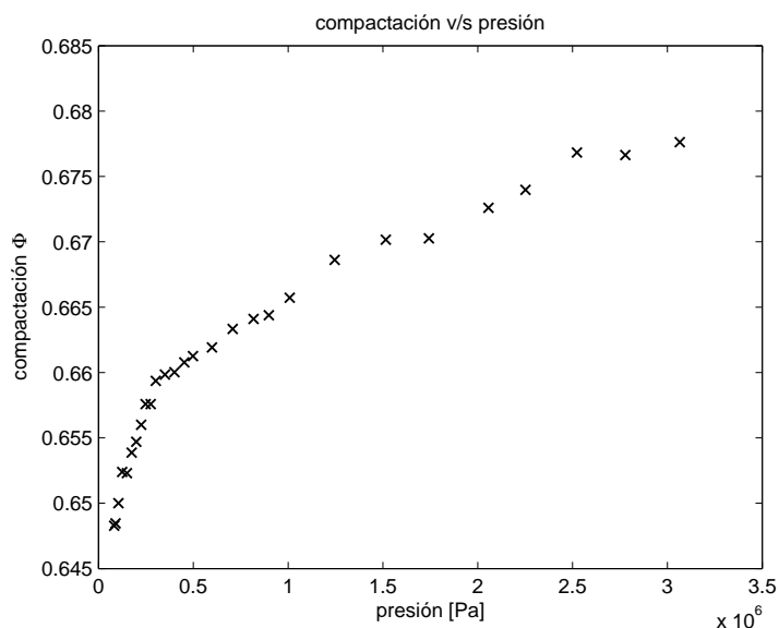
Figura 3.4: Evolución típica de la compactación \Phi según la fuerza de compresión aplicada.
