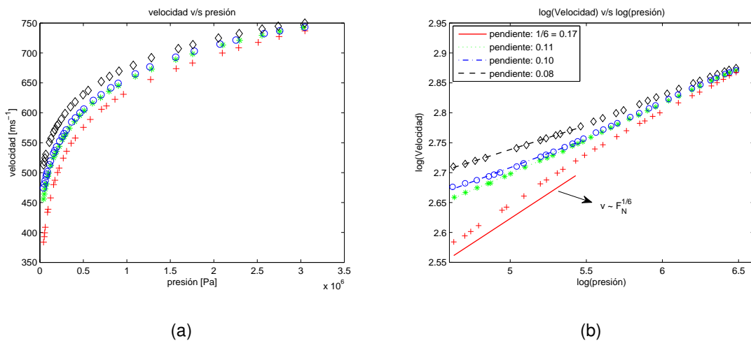
Figura 4.4: Evolución de la velocidad v de propagación de la onda en función de la fuerza F_N de compresión aplicada para un rango de 0,04 a 3MPa en el caso seco (×) comparado con aceites Rhodorsil 47V50 (*), 47V500 (o) y 47V10000 (◇). En (a) se muestra la dependencia directa entre v y F_N y en (b) en escala logarítmica.
