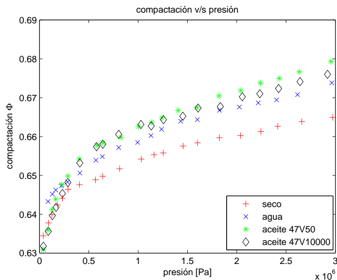
Figura 4.6: Medida de la compactación de los granos en los distintos fluidos utilizados para un rango de fuerza de compresión de 0,08 a 3MPa .
